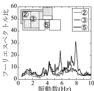
図 12 F 邸の間口方向の フーリエスペクトル比
