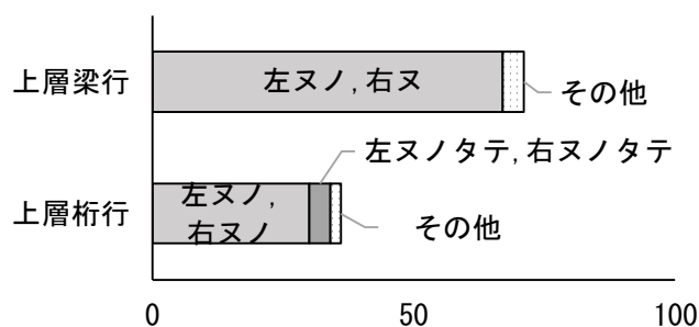
図3 上層部の緊結方法の分類（布材1本建地2本の場合）
