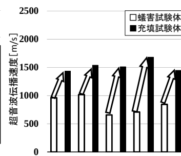
図 17 充填前後の超音波伝播速度関係
