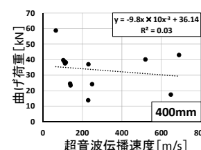
図 27 表面法（400mm）
