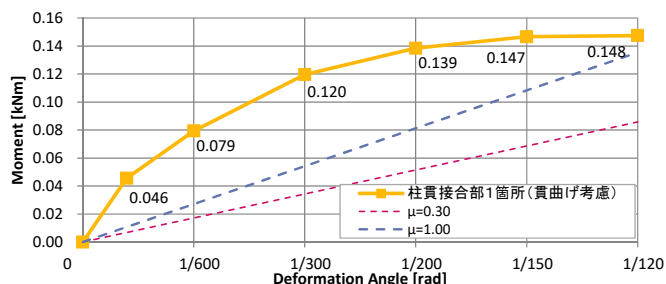
図9: 水平加力実験から導出された柱頭接合部の骨格曲線
