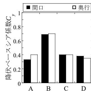
図 15 降伏ベースシア係数 C_y
