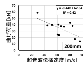
図 28 表面法（200mm）
