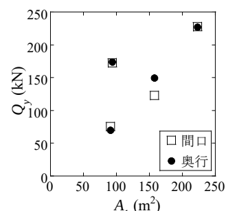
図 18 A_1 と Q_y の関係
