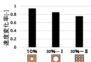
※速度変化率：穿孔後/穿孔前 図5 穿孔前後の速度変化率
