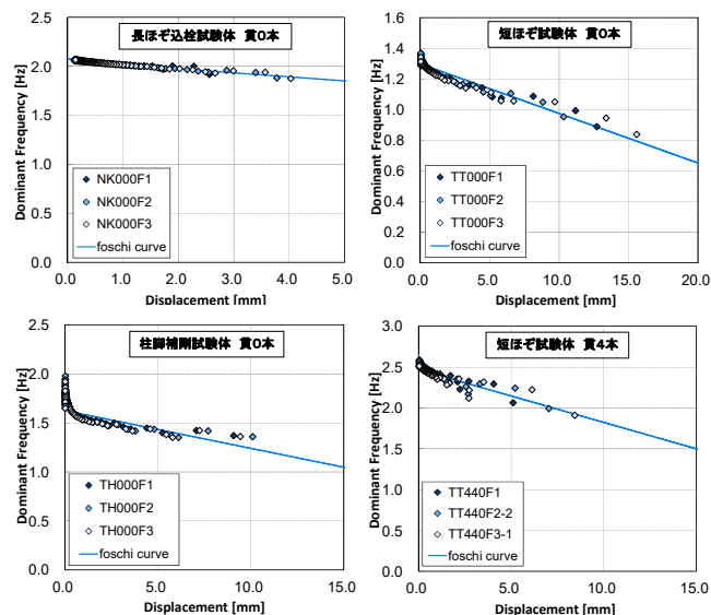
図4:軸組試験体の卓越振動数の振幅依存性と近似曲線の例(800kg)
