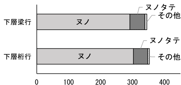
図5 下層部の接合方法の分類（布材1本建地1本の場合）
