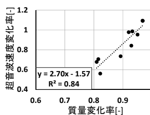
図8 超音波伝播速度と質量の変化率
