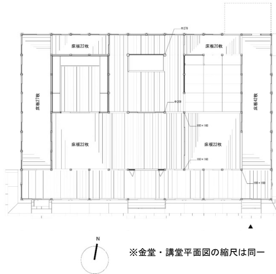
図 2：講堂平面図
