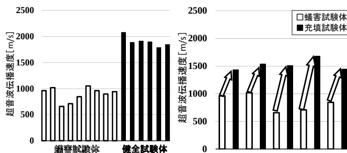
図 16 超音波速度による蟻害試験体と健全材の比較
