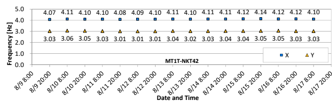
図2:同一試験体の継続的観測結果(垂壁試験体, 柱脚短ほぞ, 400kg)
