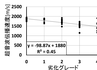
図9 超音波伝播速度と劣化グレード
