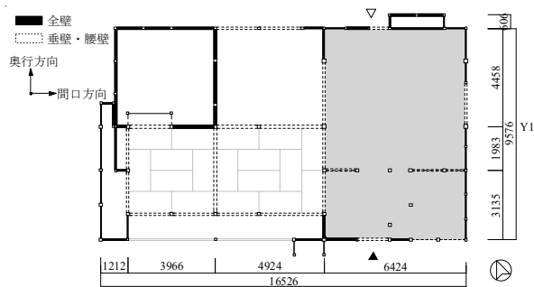
図2 平面図(A邸)
