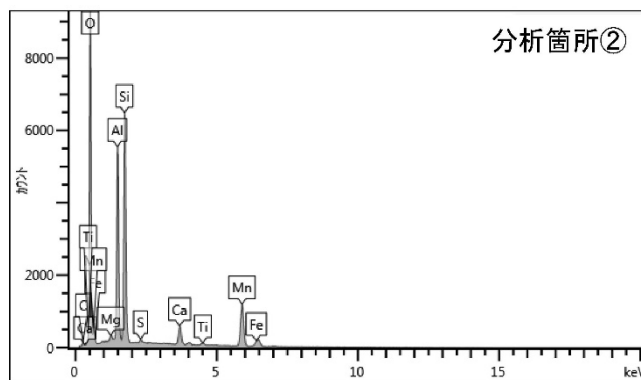
図 5 EDS による介在物 (L-1) 観察結果
