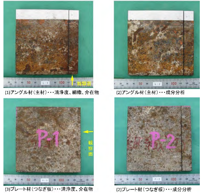
図3-1 アングルとプレートの観察用試料
