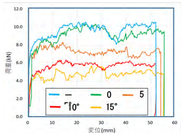
図-2 築石の各傾斜角度における押し出し荷重（摩擦抵抗）と変位の関係 2)
