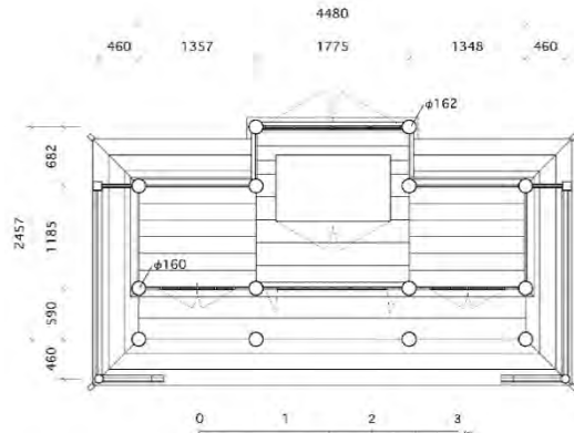
図8 那古寺宮殿の平面図（単位：mm）
