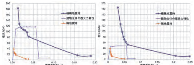
(a) 夏季・桁行方向
