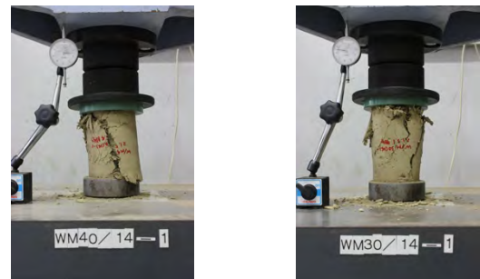
水土比 40% 14日
