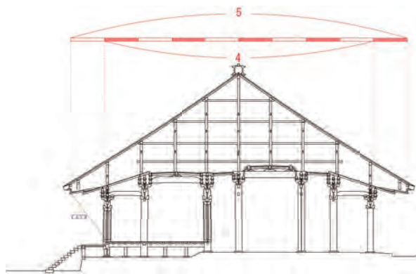
図3-5 延暦寺転法輪堂の軒比率と禪墨
