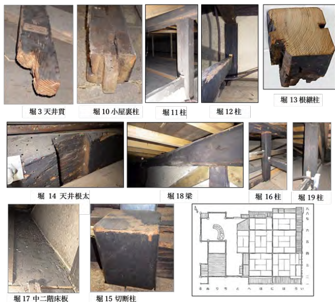
図1 資料写真および堀家住宅平面解体番付
