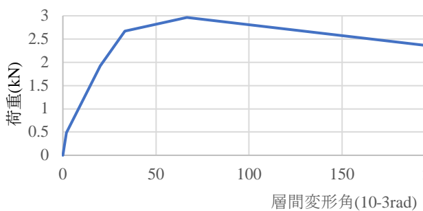
図9 接合部の解析モデル
