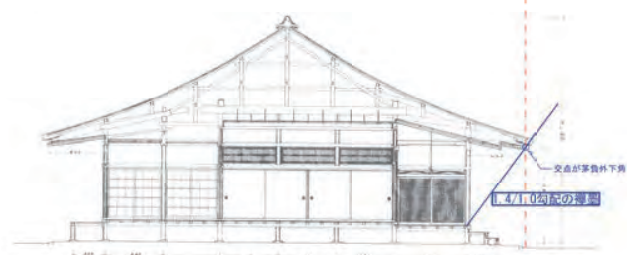
図 2-4 竜吟庵方丈の禪墨による軒の高さの決定
