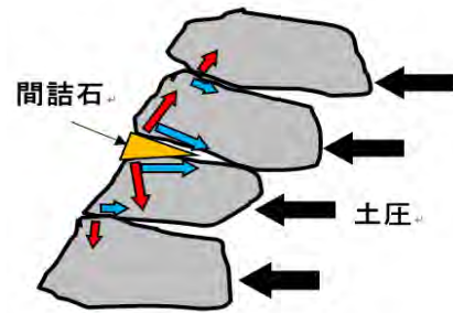
図-2 間詰石の摩擦抵抗機能
