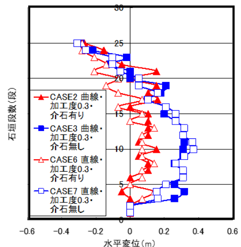
図-6 臙介石の有無による石垣のはらみ出し量の比較
