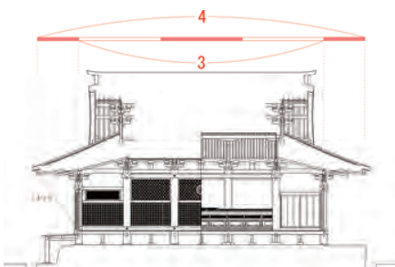
図3-3 西明寺本堂の軒比率と禪墨
