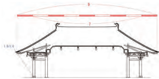
図3-1 唐招提寺金堂の軒比率と禪墨
