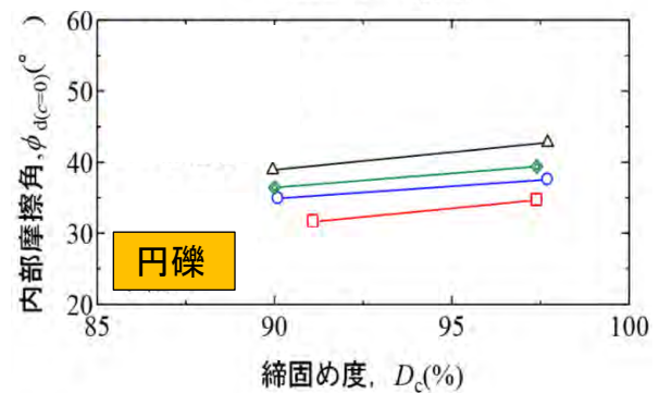
図-8 角礫と円礫の締め固め度と摩擦抵抗 3)
