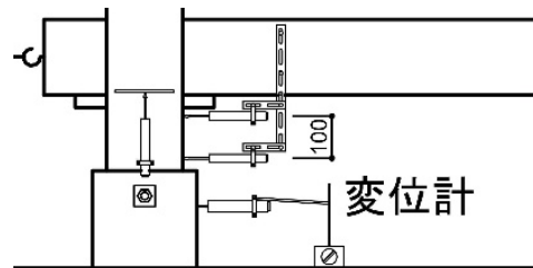
図4 柱脚拡大図
