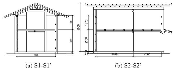
図2 N邸断面図
