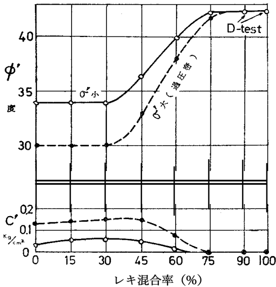
図-9 礫混合率による摩擦角 ( \phi ) と粘着力 ( c' ) の変化 4)
