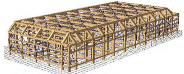
図11 解析モデル
