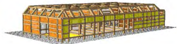
図12 解析結果の一例（加振後の損傷状況）
