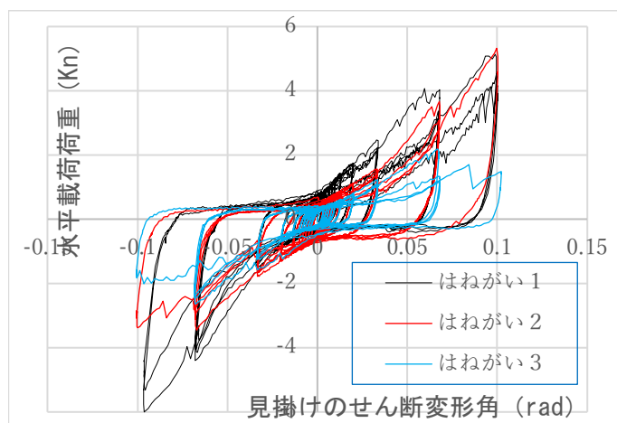
図 8 はねがいの復元力特性
