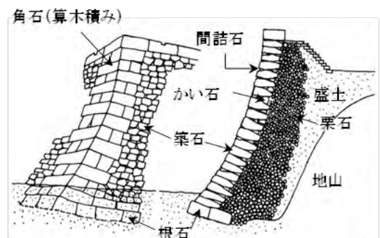
図-1 城郭石垣の構造と各部の名称 2)
