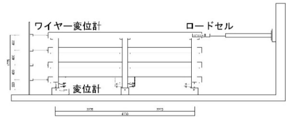
図3 変位計設置図
