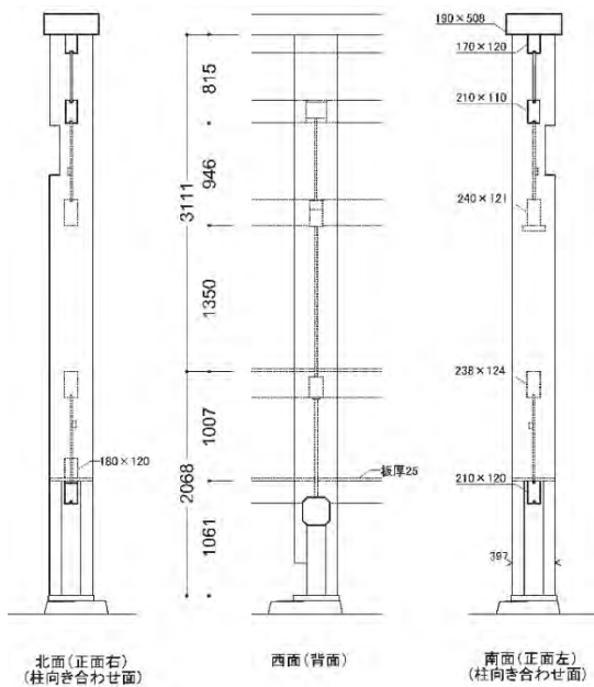
図5 大山寺宮殿の内部柱の痕跡図(単位: mm)
