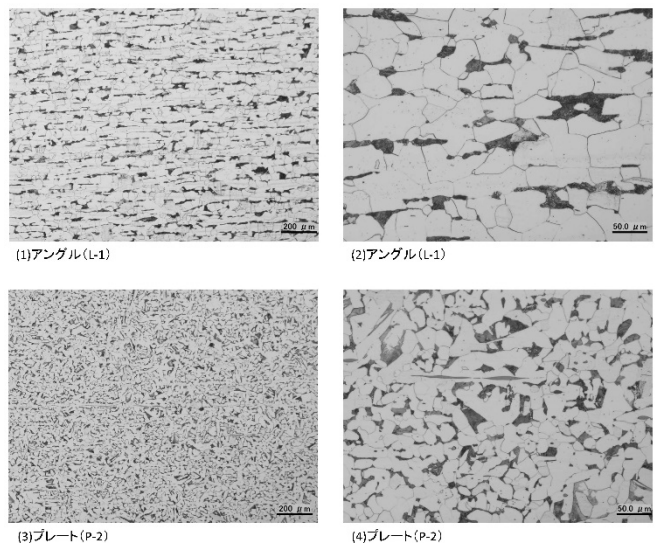
図4-1 アングルとプレートの金属組織観察結果
