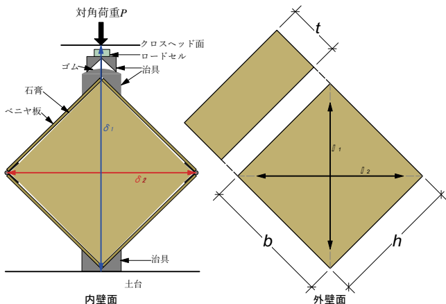
図9 加力システムと変位の計測位置
