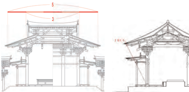
図3-2 平等院鳳凰堂身舎軒の軒比率と禪墨
