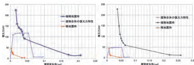
(c) 冬季・桁行方向
