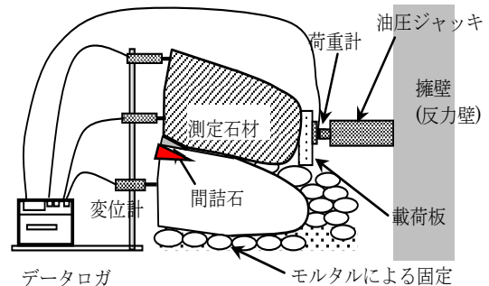
図-2 間詰石の摩擦抵抗機能
