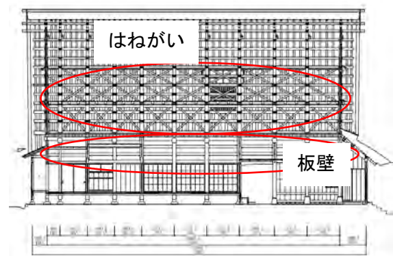
図 2 断面図及び構造要素の位置
