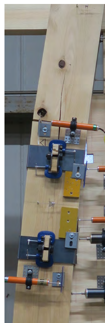
< 試験体 5 >
