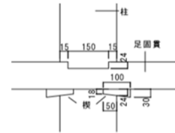
(f) 内法貫・足固貫
