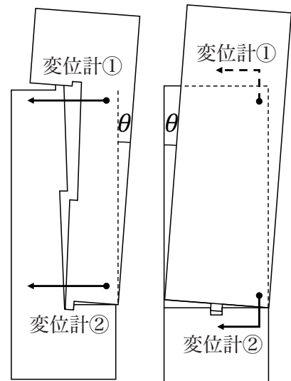
図5 継手の回転角の計測方法 (左：弱軸方向／右：強軸方向)
