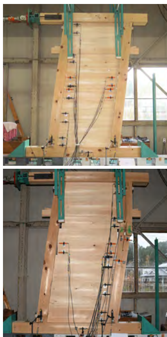
写真 1 1/10\text{rad} 時の様子 (上: 試験体 1 / 下: 試験体 4)
