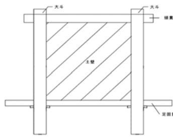
(b) 試験体
