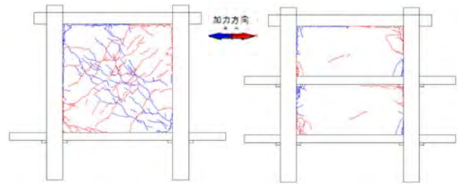
(a) 試験体II
