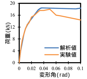
(d) 試験体IV
