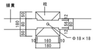
(c) 頭貫
