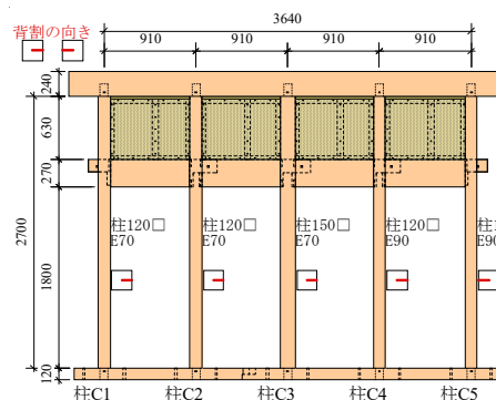
図1 試験体
