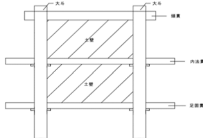
(d) 試験体
