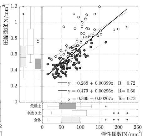
(c) 弾性係数と圧縮強度
