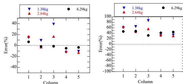
(a) 密度 (b) 曲げヤング係数
