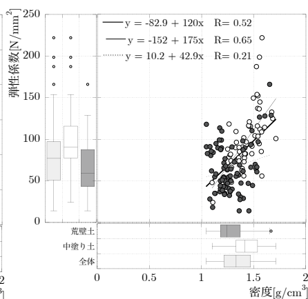
(b) 密度と弾性係数
