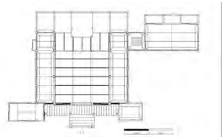
図6 発軫閣 平面図
