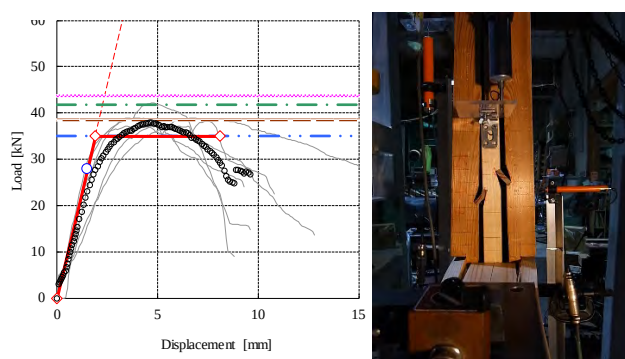
図2 車知栓接合部の引張挙動と変形の様子
