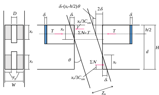
図3 両引き接合部の回転抵抗力学モデル
