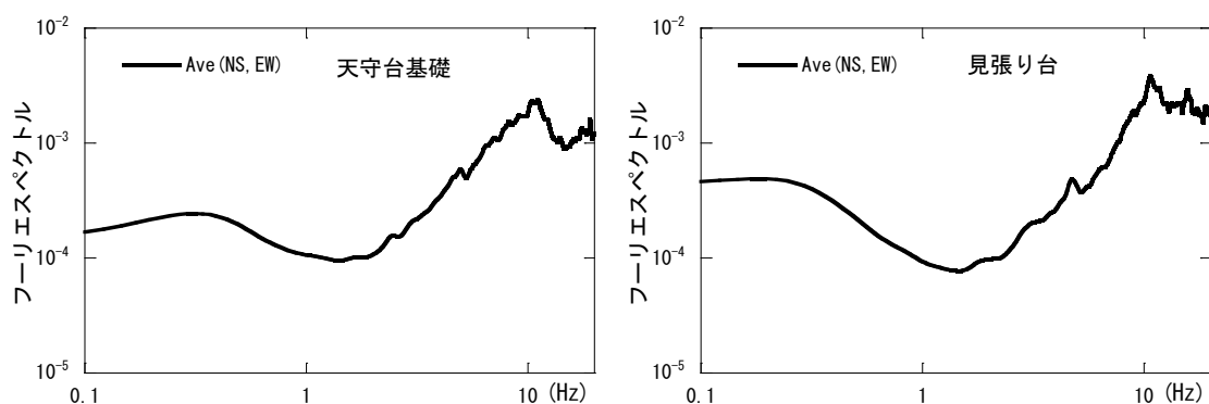
図3 平均化した水平成分のフーリエスペクトル ( H_F 、 H_G )
