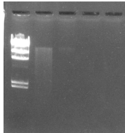
図4 抽出DNAの電気泳動図
