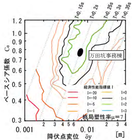
図-6 Case4 (b)補強鉄骨・耐震プレート増設
