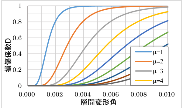
図-3 損傷係数Dと層間変形角の関係
