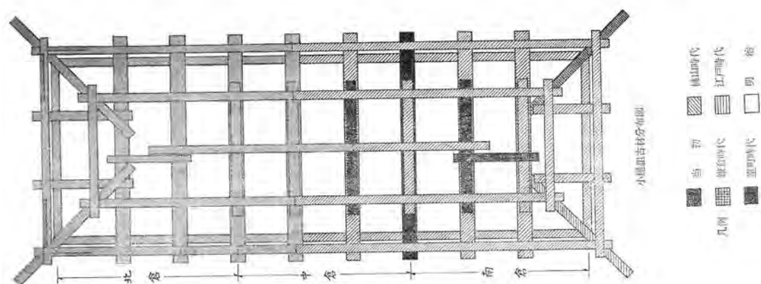
図1 法隆寺綱封蔵の小屋組古材（出典：修理工事報告書）
