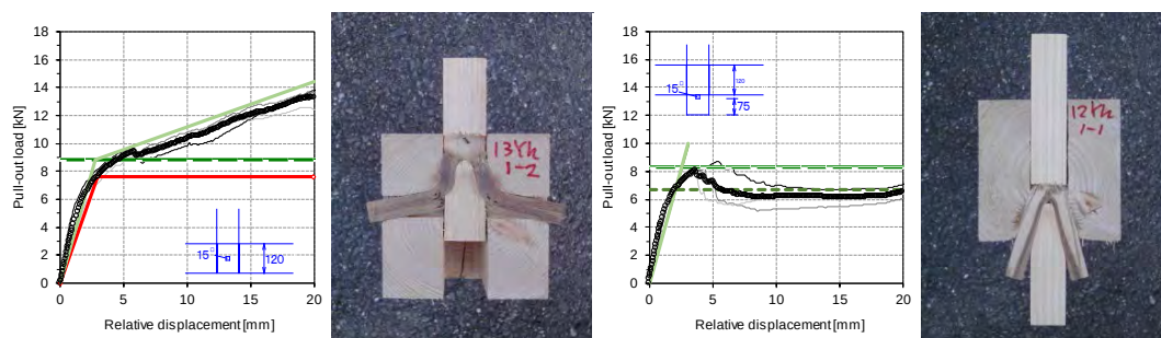
図1 込栓・鼻栓接合部の引張挙動と変形の様子
