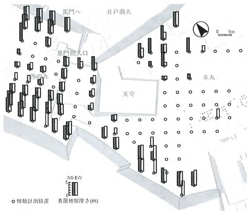
図2 表層地盤厚さの推定分布
