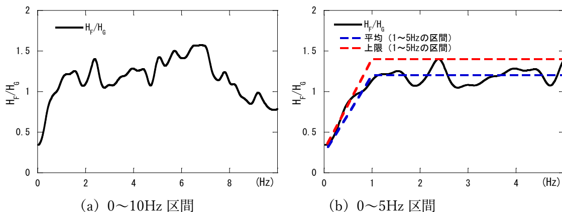
図4 地山に対する天守台基礎の水平成分フーリエスペクトル比 ( H_F/H_G )
