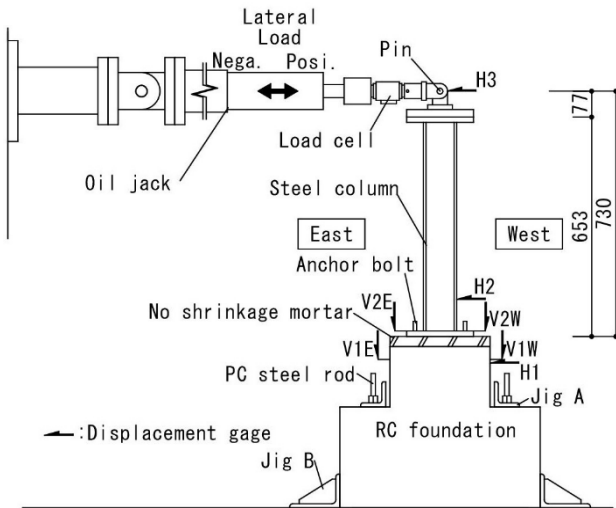
Fig. 2 Setup
