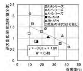
図 19 食害率 -耐力変化率
