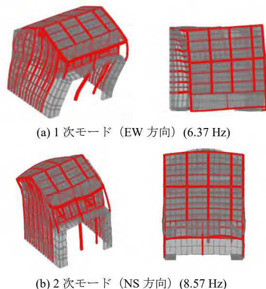
図3 振動モード
