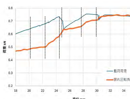
図 19 C の捩れ回転角と載荷荷重の変化
