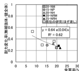
図 18 食害率 -耐力変化率
