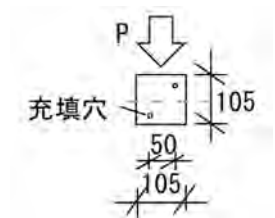
図10 試験体概要
