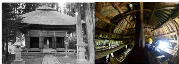
図1 (左) 青森県八戸市に所在する清水寺観音堂外観(左)・小屋裏(右)
