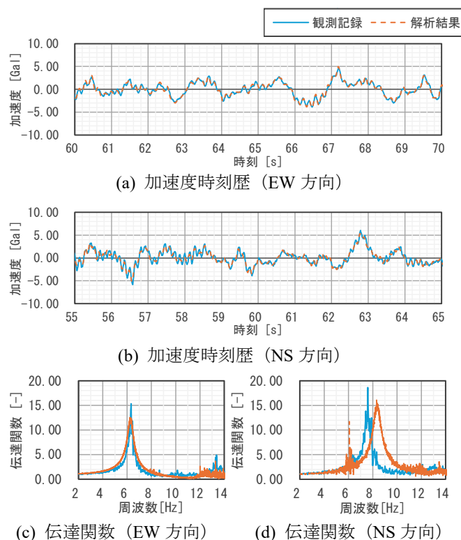
図4 地震観測点の時刻歴および伝達関数
