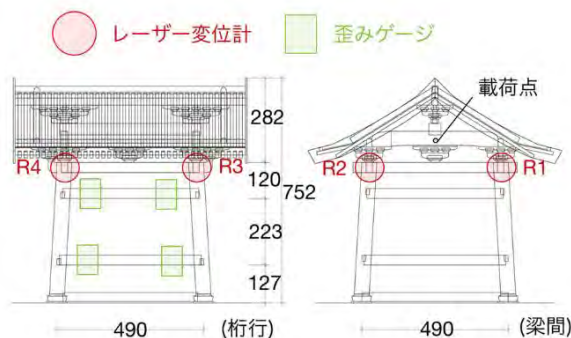
図 16 模型寸法および荷重装置・計測機器の設置位置
