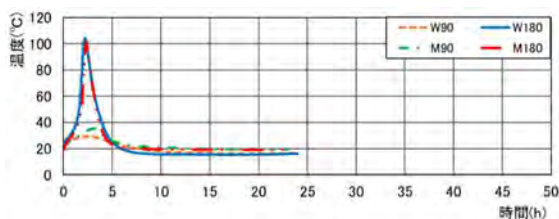
図3 試験結果(充填回数1回)
