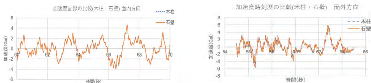
図 1 地震動観測結果
