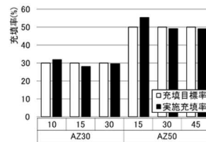
図11 充填率
