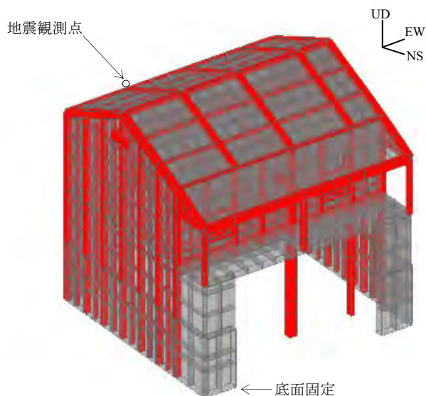
図2 解析モデル
