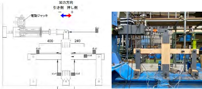
図3 実験のセットアップ
