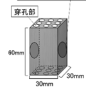
図5 試験体概略図
