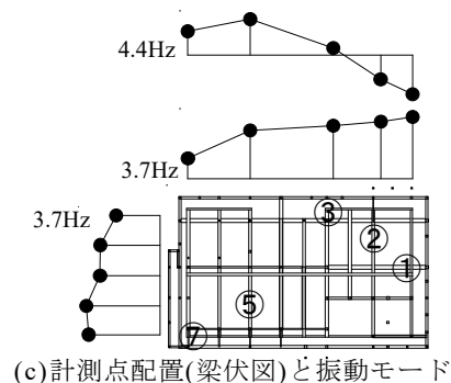
(c) 計測点配置(梁伏図)と振動モード
