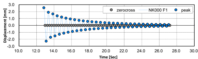
図3: 人力加振試験による自由振動波形例 (FA2, 長ほぞ込栓, 800kg, 貫0本)
