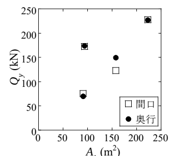
図 18 A_1 と Q_y の関係
