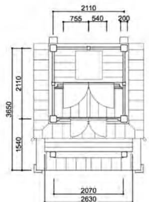
図9 平面図
