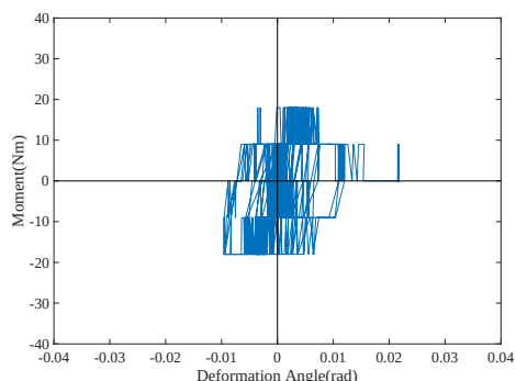
図 13 モーメントー変形角関係 (タテ型)
