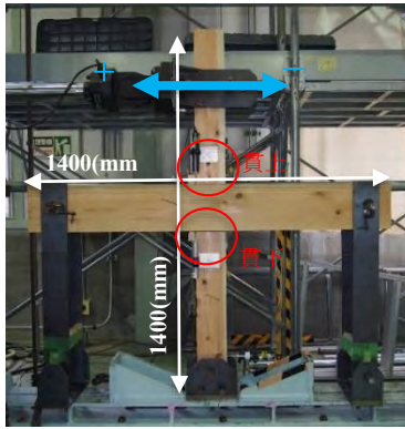
図 7 荷重装置
