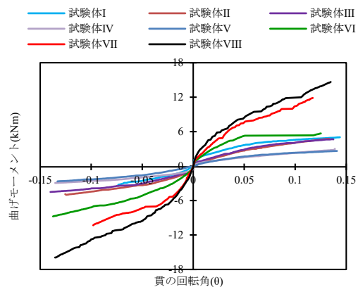
図5 試験体ごとの比較
