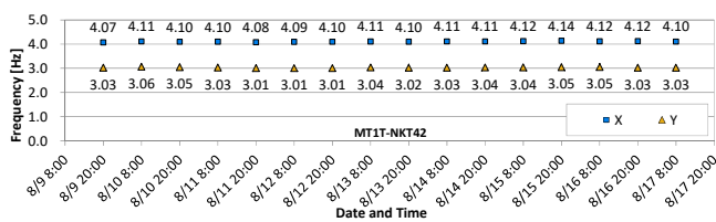
図2: 同一試験体の継続的観測結果（垂壁試験体、柱脚短ほぞ、400kg）
