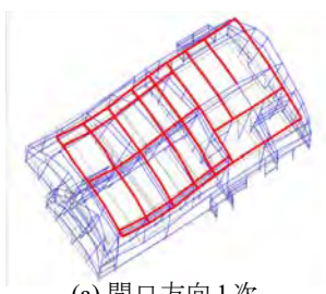
図6 固有振動モード(3Dモデル)
