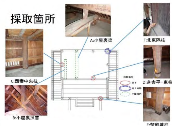
図 4 試料採取箇所
