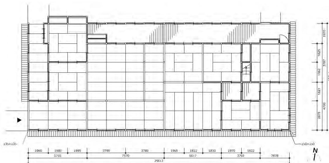
図3 客殿平面図
