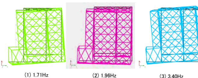
図14: 月光殿の解析モデルの固有値解析結果
