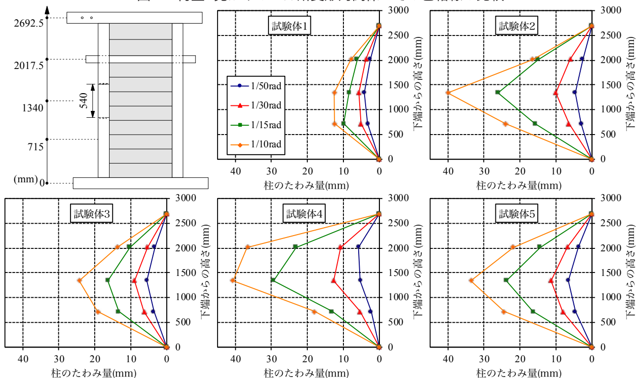
図3 柱のたわみ量の比較と計測点の位置
