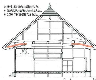
図7 正善寺本堂 梁行断面図 S=1:300
