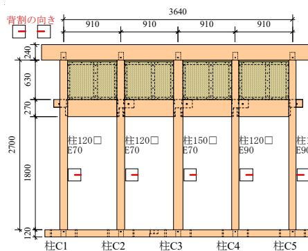
図1 試験体
