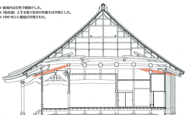
図6 吉祥寺本堂 梁行断面図 S=1:300
