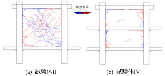
図4 1/15rad 時における土塗壁の破壊性状
